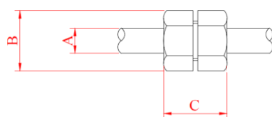
Priama spojka
